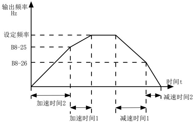
图 6-16 加减速时间切换示意图
