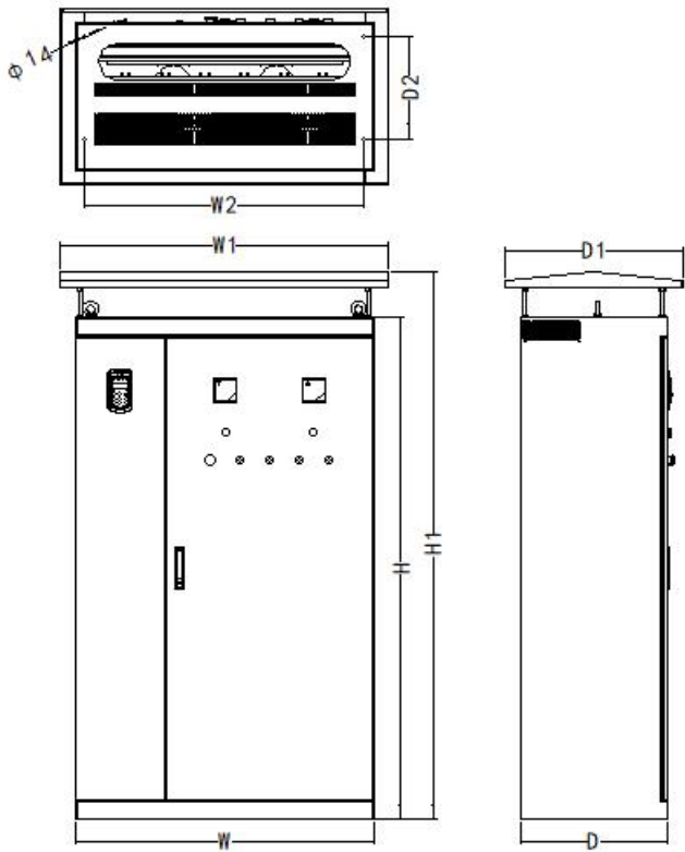
3. G550~G630KW 金属外壳变频器外形及尺寸示意图
