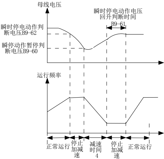
图 6-22 瞬时停电动作示意图
