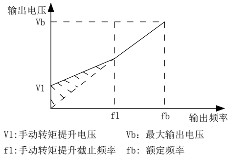
图 6-2 手动转矩提升示意图
