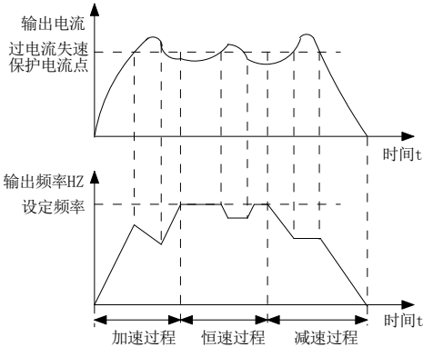
图 6-21 过流失速保护示意图
