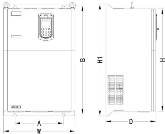
3. G550~G630KW 金属外壳变频器外形及尺寸示意图
