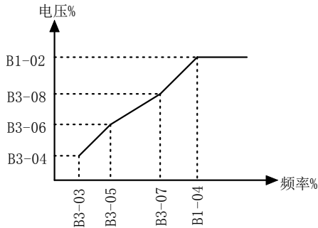
图 6-3 多点 V/F 曲线设定示意图
