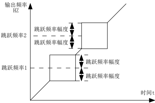
图 6-11 跳跃频率示意图
