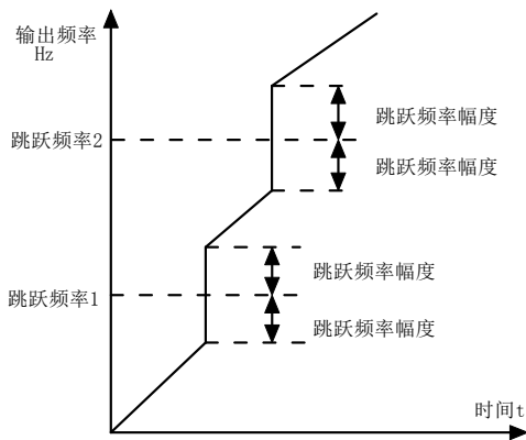
图 6-15 加减速过程中跳跃频率有效示意图
